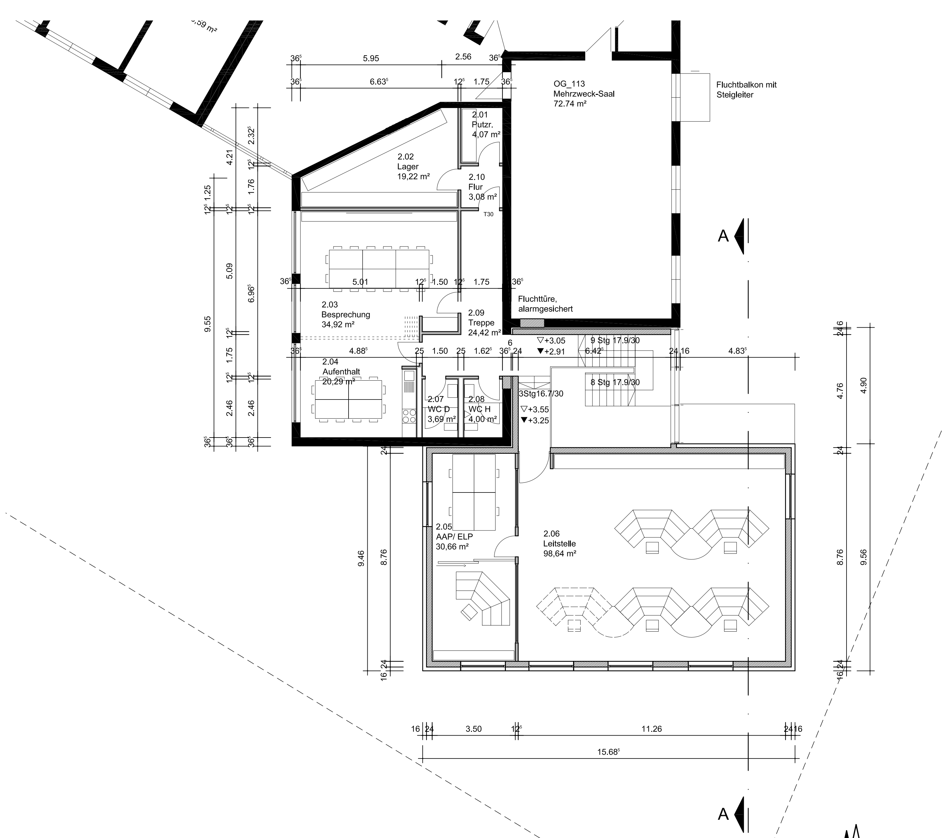
Grundriss Obergeschoss
