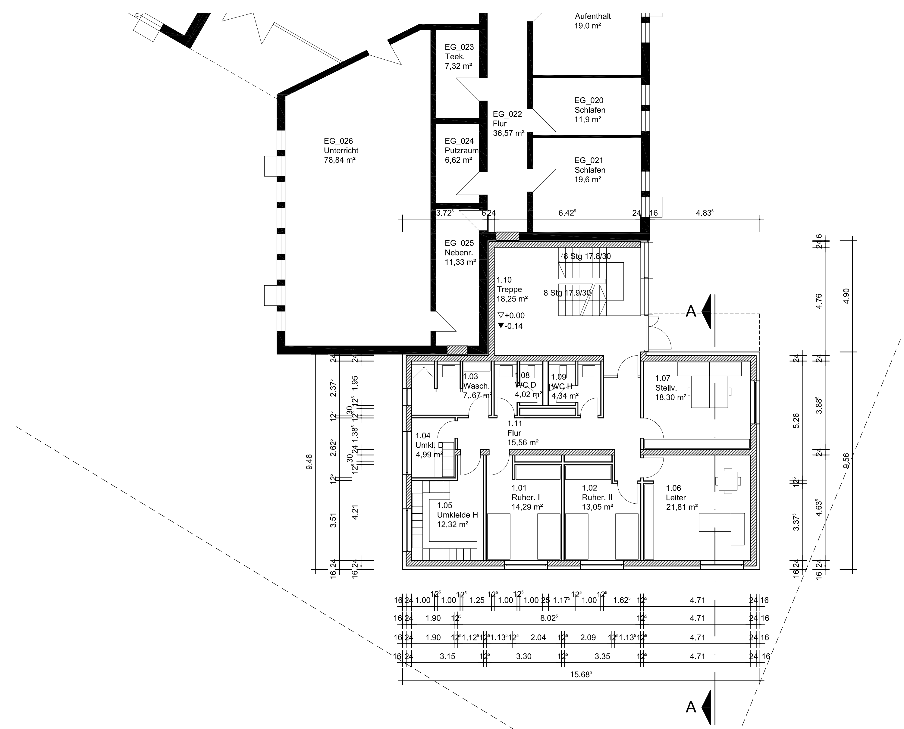
Grundriss Erdegesschoss
