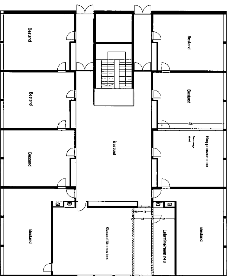
GRUNDRISS VERBINDUNGSRAMPE IM BEREICH DES 1. OBERGESCHOSSES
