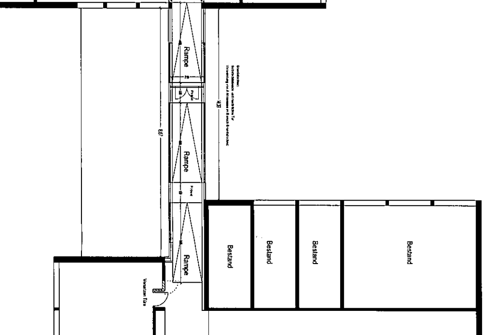
BAUABSCHNITT 606r
